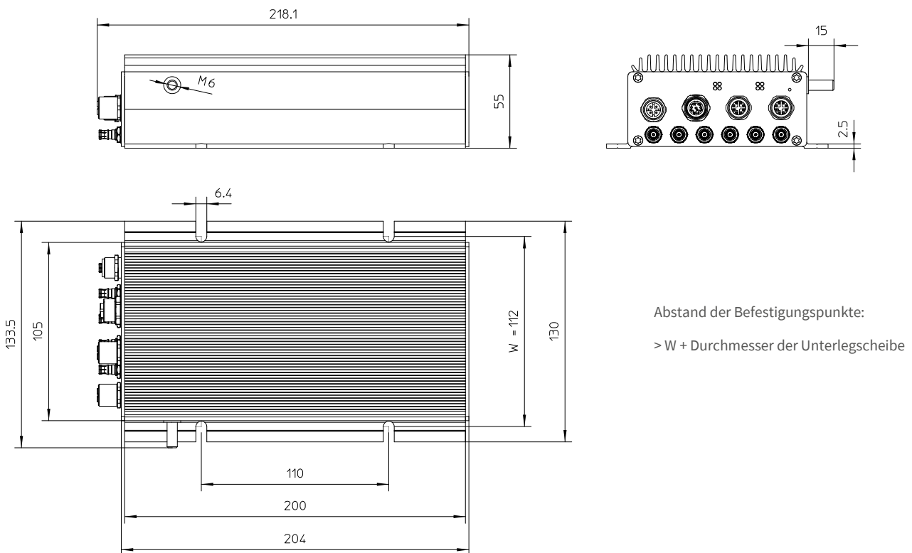
Figure 5 Abmessungen des CyBox AP 2- und CyBox LTE 2-Gehäuses
